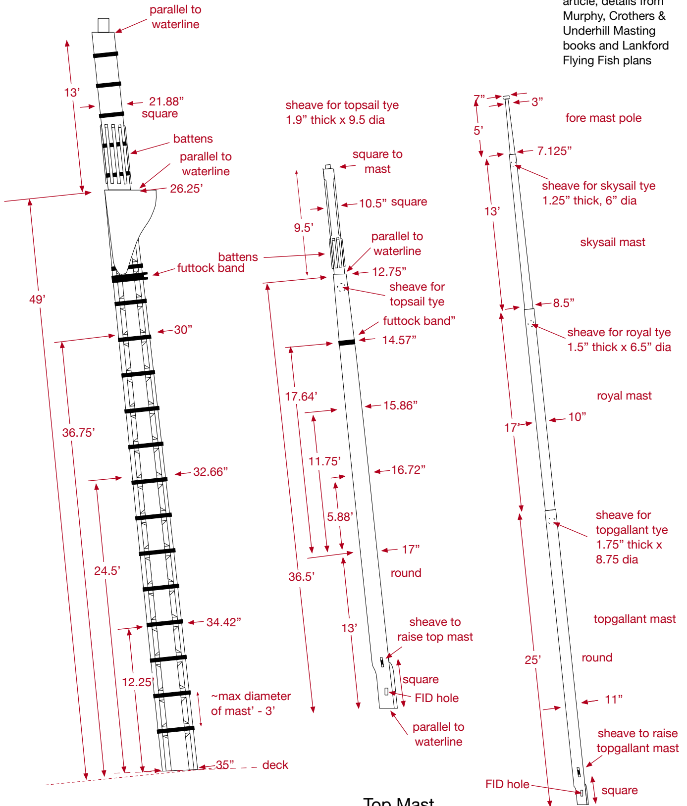
Topgallant Mast
